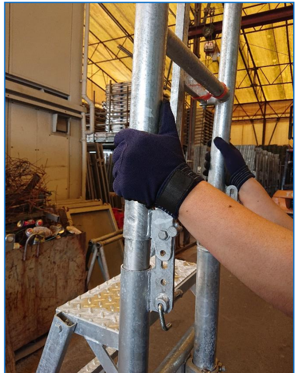
⑩手摺部組立
