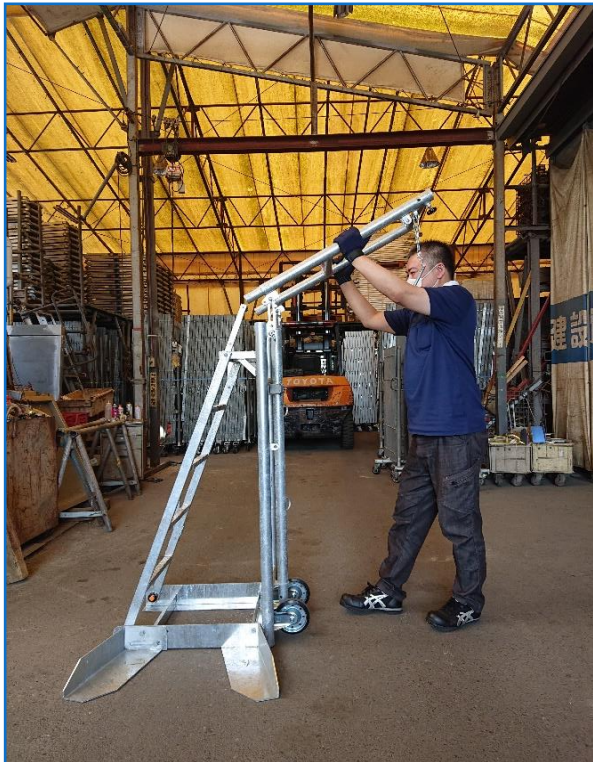
⑨支柱中間部組立
