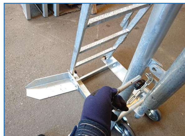
⑥支柱中間部ピン抜き
