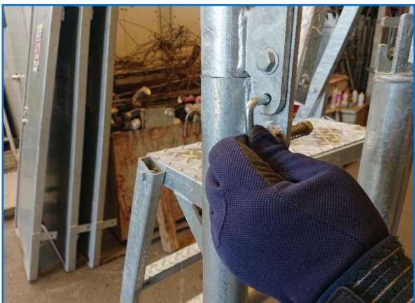
⑪手摺部組立
